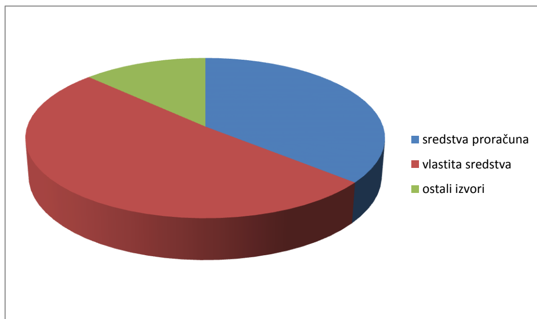
Grafikon 1. Prikaz udjela sredstava za programe javnih potreba u kulturi u 2014. godini
